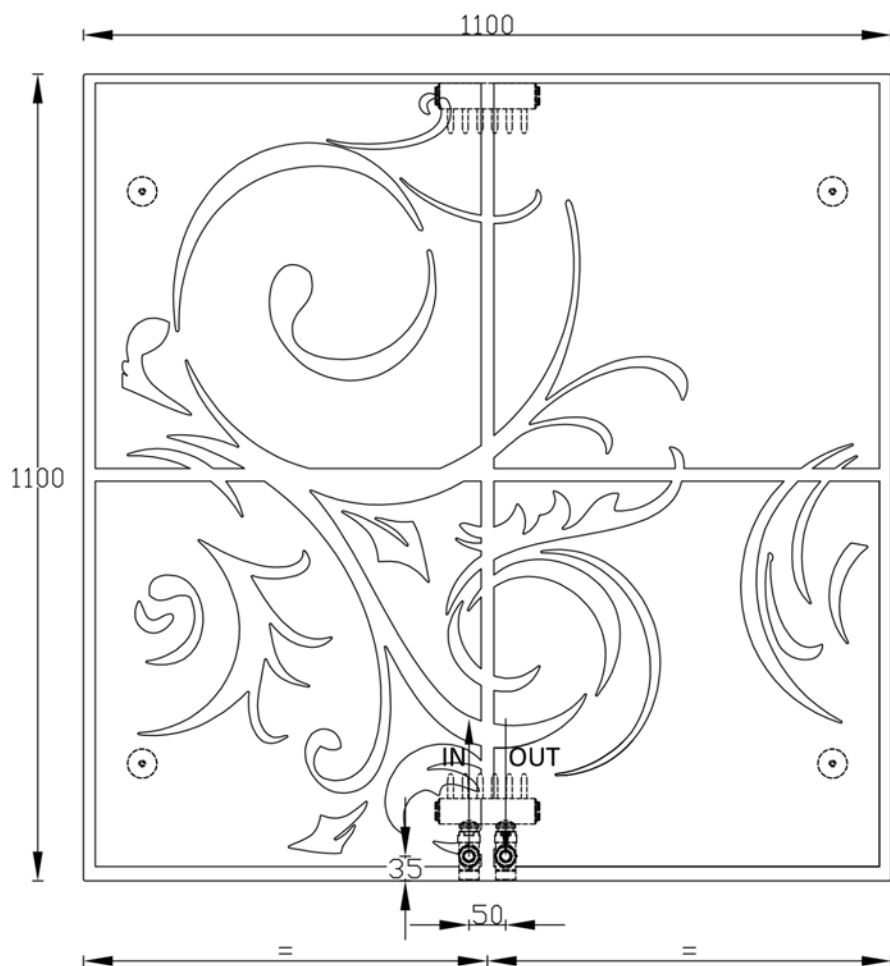
Vista frontale - Front view - Vue de face
