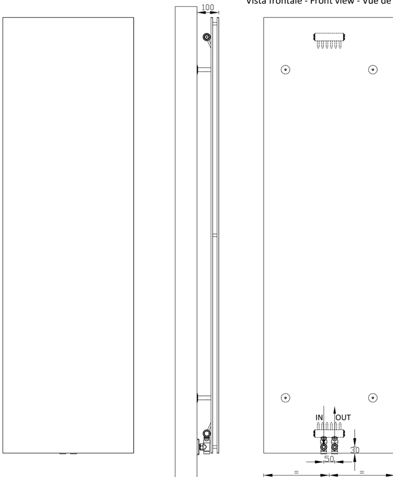
Vista frontale - Front view - Vue de face
